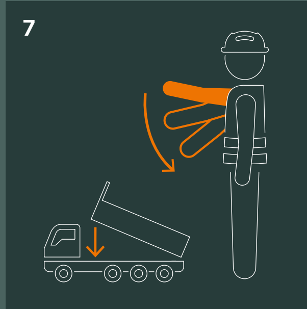
Senken des Kippers
